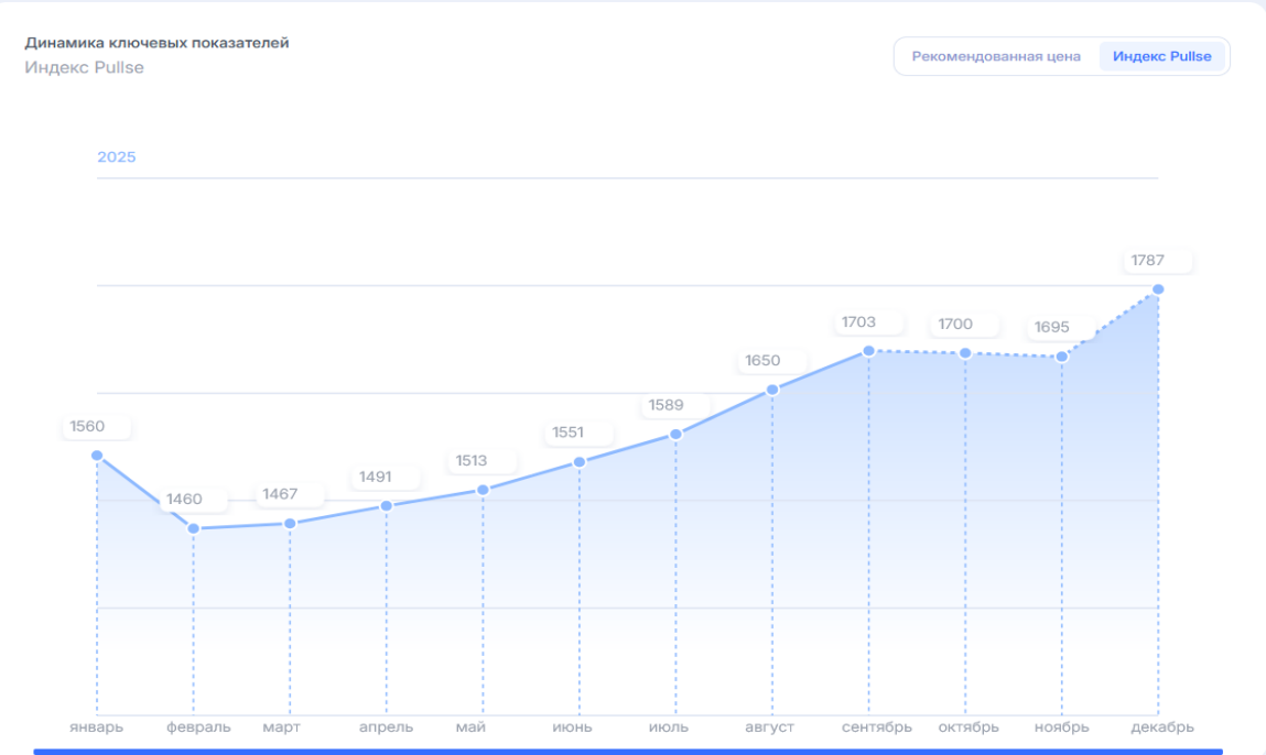
Рисунок 3 – Вкладка «Прайсинг»
