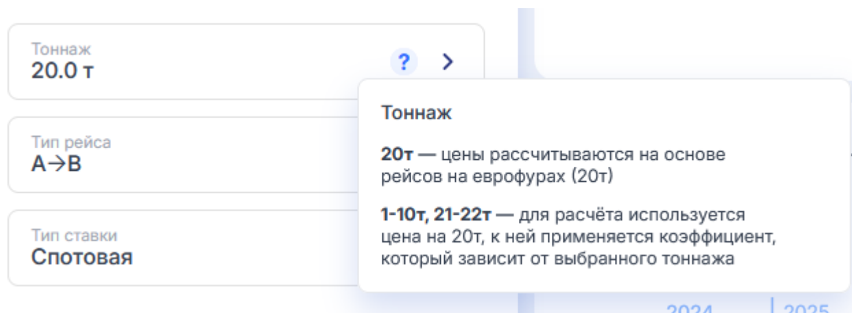
Рисунок 14 – «Тоннаж», подсказка
