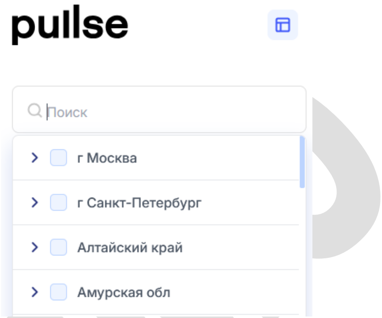
Рисунок 7 – Окно поиска
